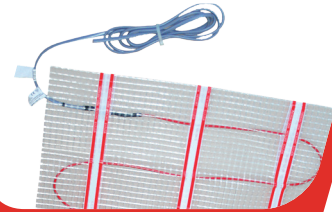
Elektro- Fußbodenheizung
